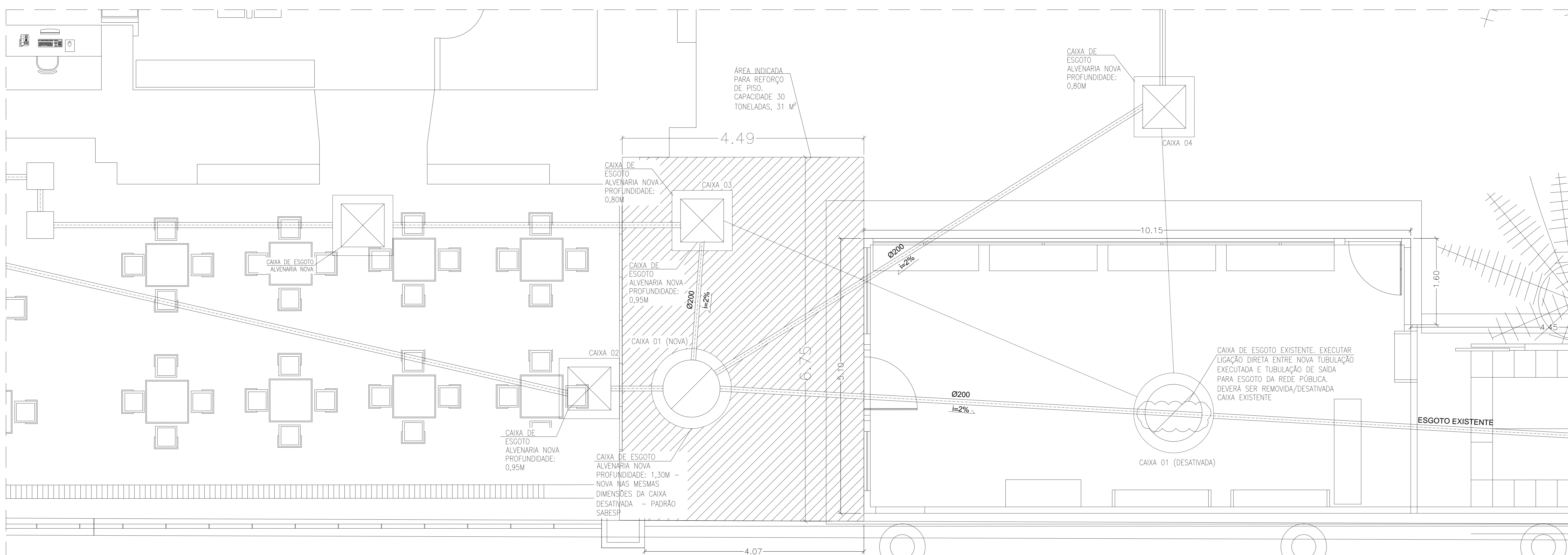
AMPLIAÇÃO DE TRECHO NOVO ESCALA 1:50
